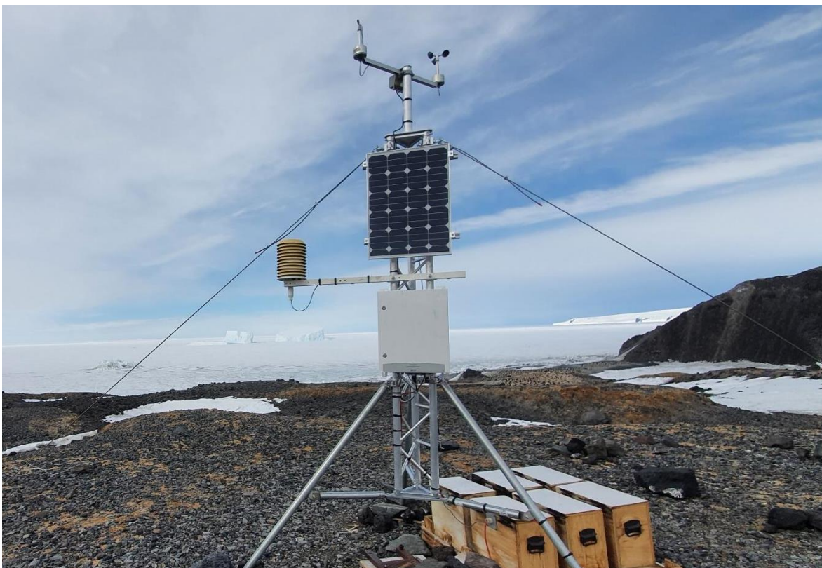
Osservatorio meteo-climatologico installato presso la Stazione Mario Zucchelli
