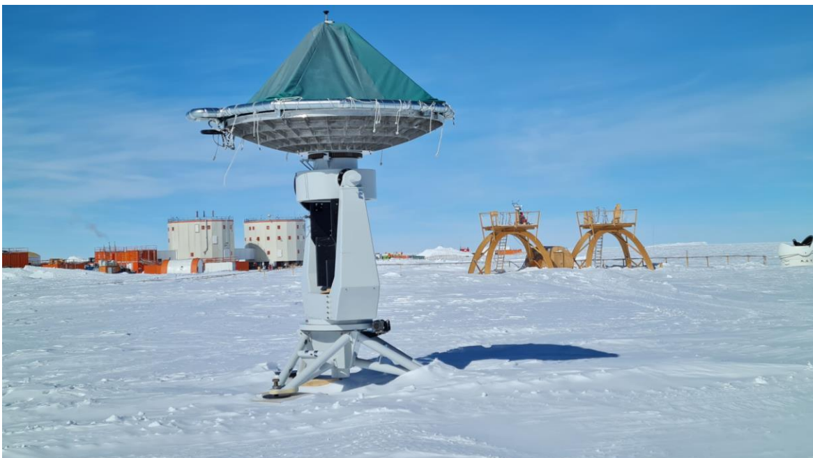
COCHISE - In primo piano, Cochise, un telescopio di 2,6 metri di diametro dedicato ad osservazioni di cosmologia in banda millimetrica e sub-millimetrica installato a Dome-C nei pressi della Stazione Concordia.
